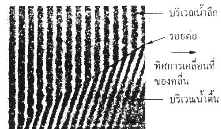
รูปที่ 2 การหักเหเมื่อหน้าคลื่นตกกระทบไม่ตั้งฉากกับผิ্বরอยต่อ
